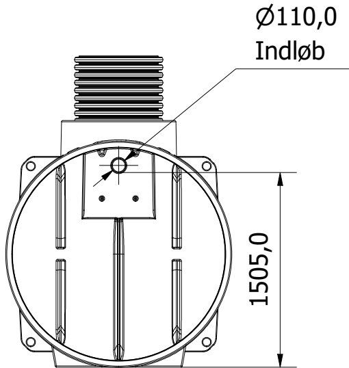
Left
