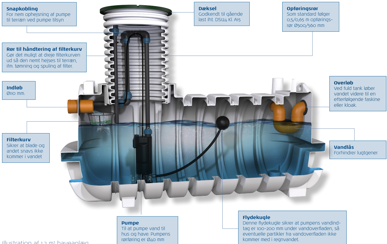
Illustration af 1,2 m³ haveanlæg
